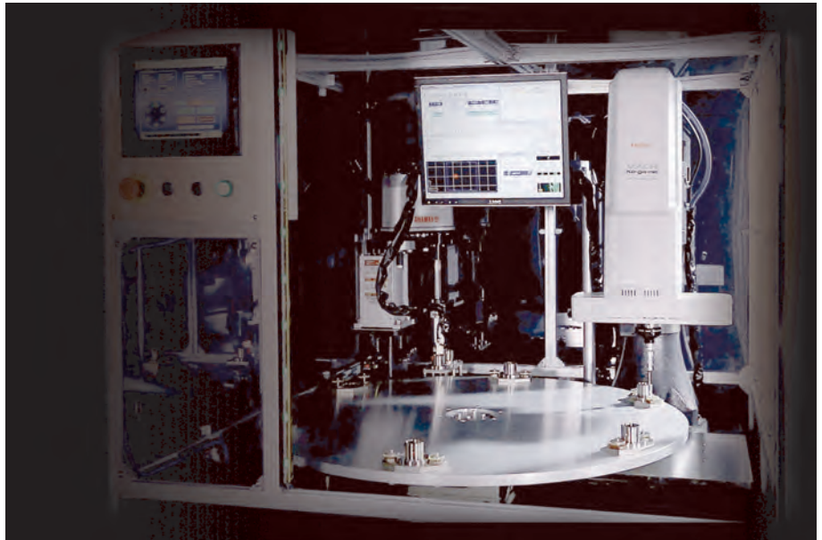
Применение КИМ МАСН Ко-га-ме в производственной линии
