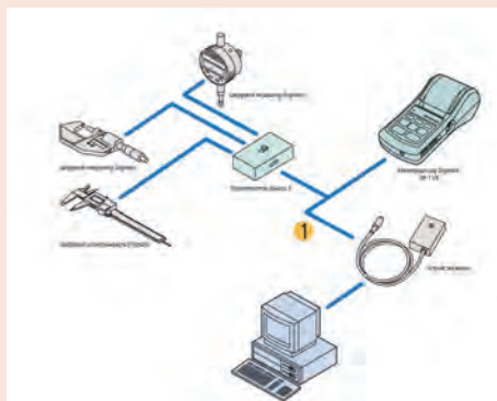
1 - кабель 936937 (1 м), 965014 (2 м)
